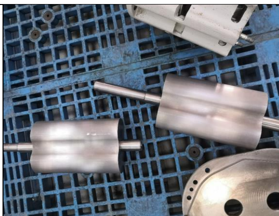
清洗打磨后的转子
