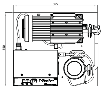
装有XDD1前级泵的T-Station 75D
