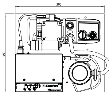
装有E2M1.5前级泵的T-Station 75W
